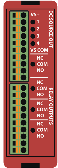
EZRPL-IO-4DCOP4RLO
